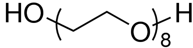
Polyethylenglycole
