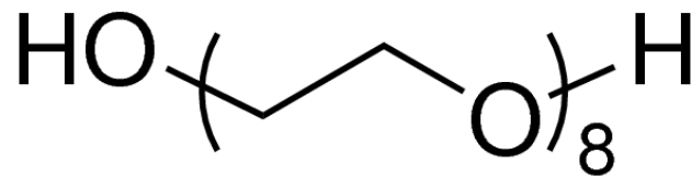
Polyethylenglycole
